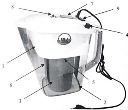
Рис. 1 - Общий вид электроактиватора
